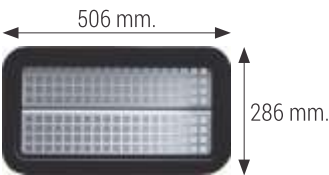
Ventana de chapa perforada. Dimensiones: 402 x 193 mm. Ventilación: 0,0342 m².
