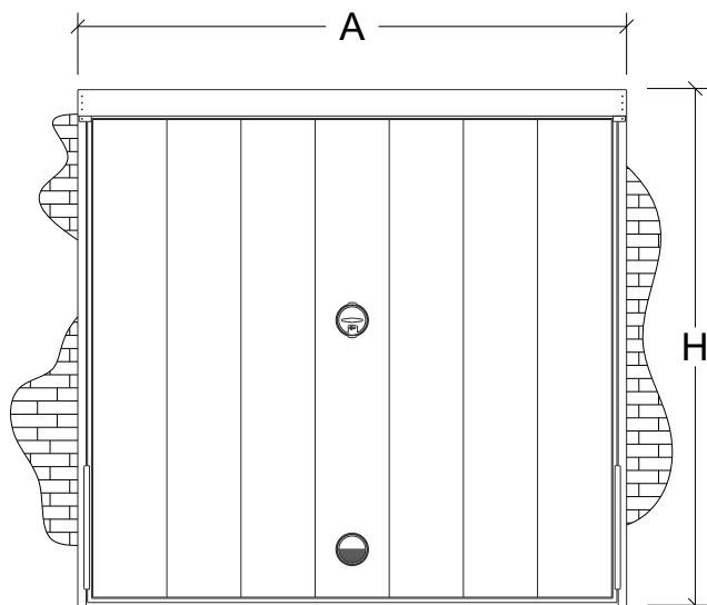
Fig. 1- Detalle de alzado de Puerta Standard Lama Lisa
