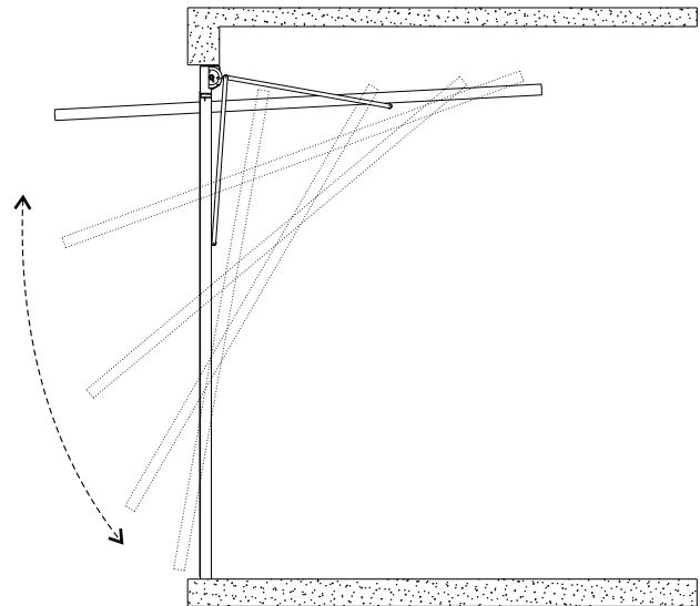
Fig. 2- Detalle de sección vertical de Puerta Standard
