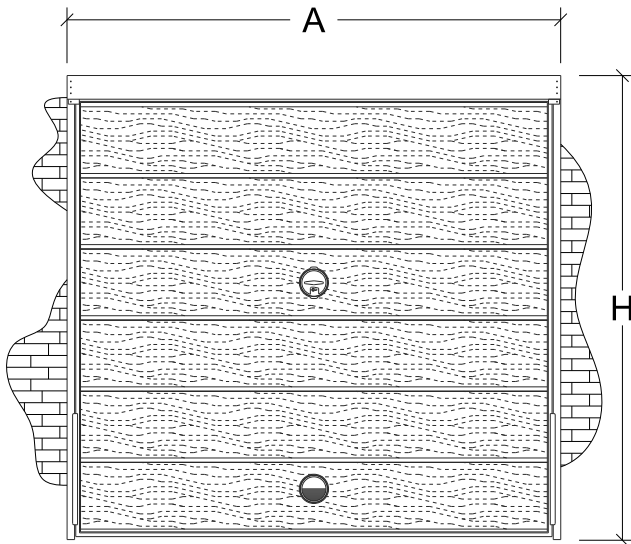
Fig. 1- Detalle de alzado de Puerta Standard Imitación Madera
